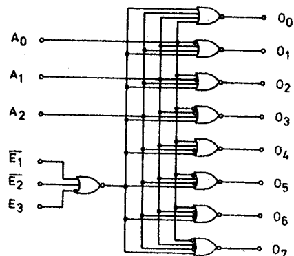
Schemat logiczny
